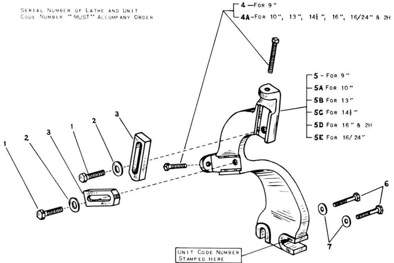
REGULAR FOLLOWER REST FOR 9", 10", 13", 14½", 16", 16/24" & 2H
